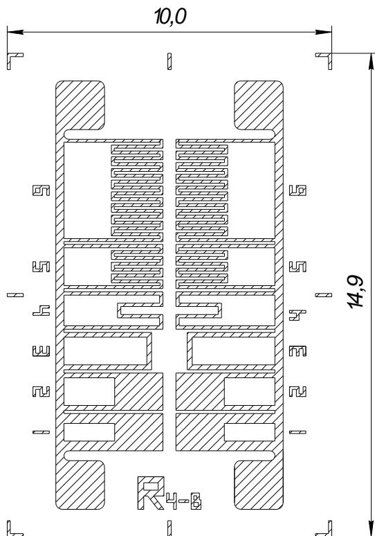
Резистор R_{ч(в)}
